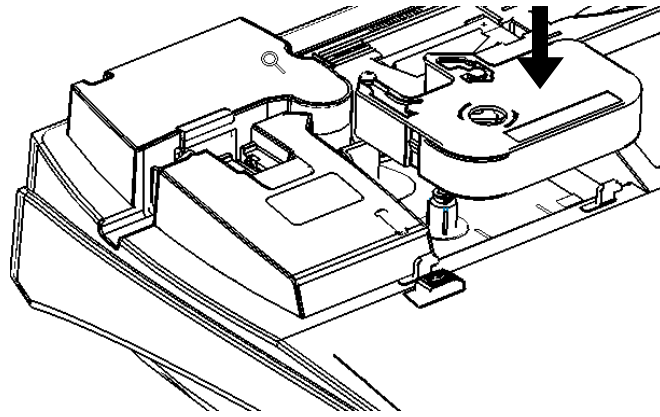
色带盒安装示意图
